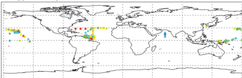
b Fe(II) / Fe total %, coarse
